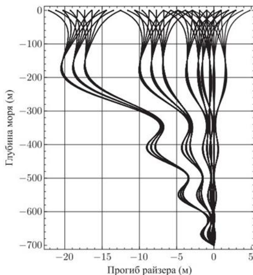
Рисунок 1 – Прогиб райзера
