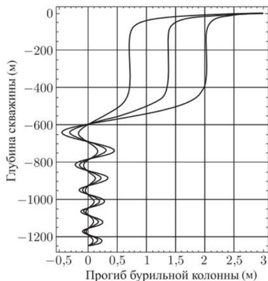
Рисунок 2 – Прогиб буровой колонны
