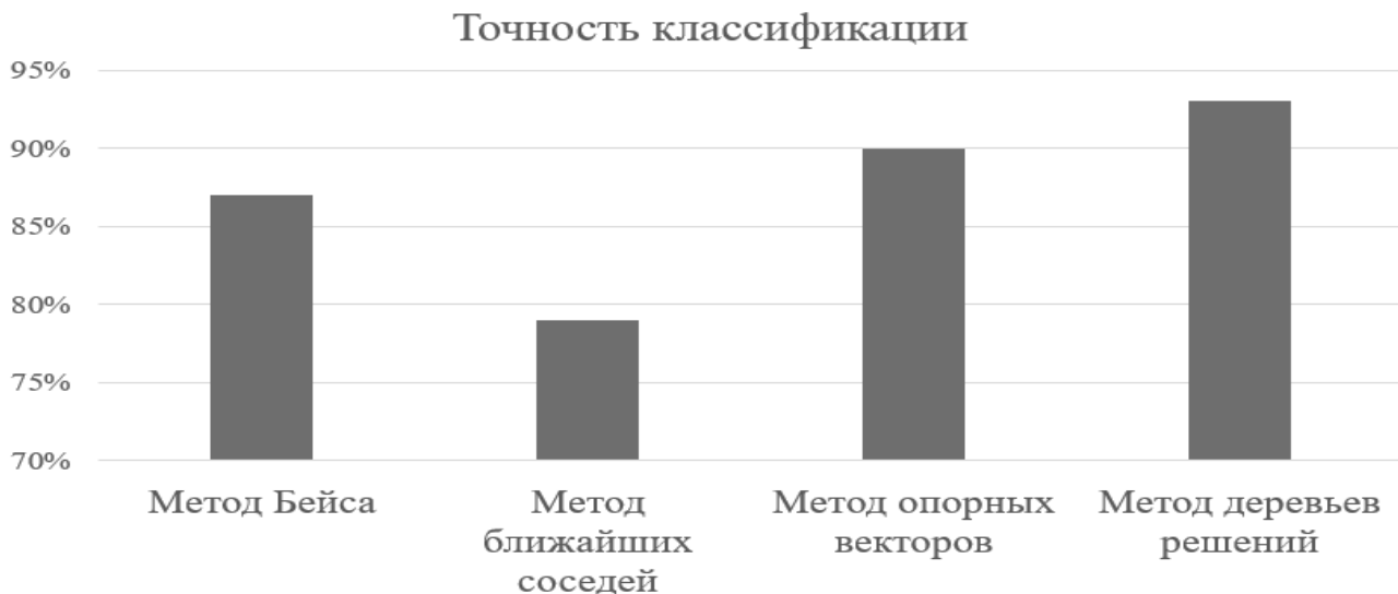
Рисунок 6 – Точность классификации сравниваемых методов.
