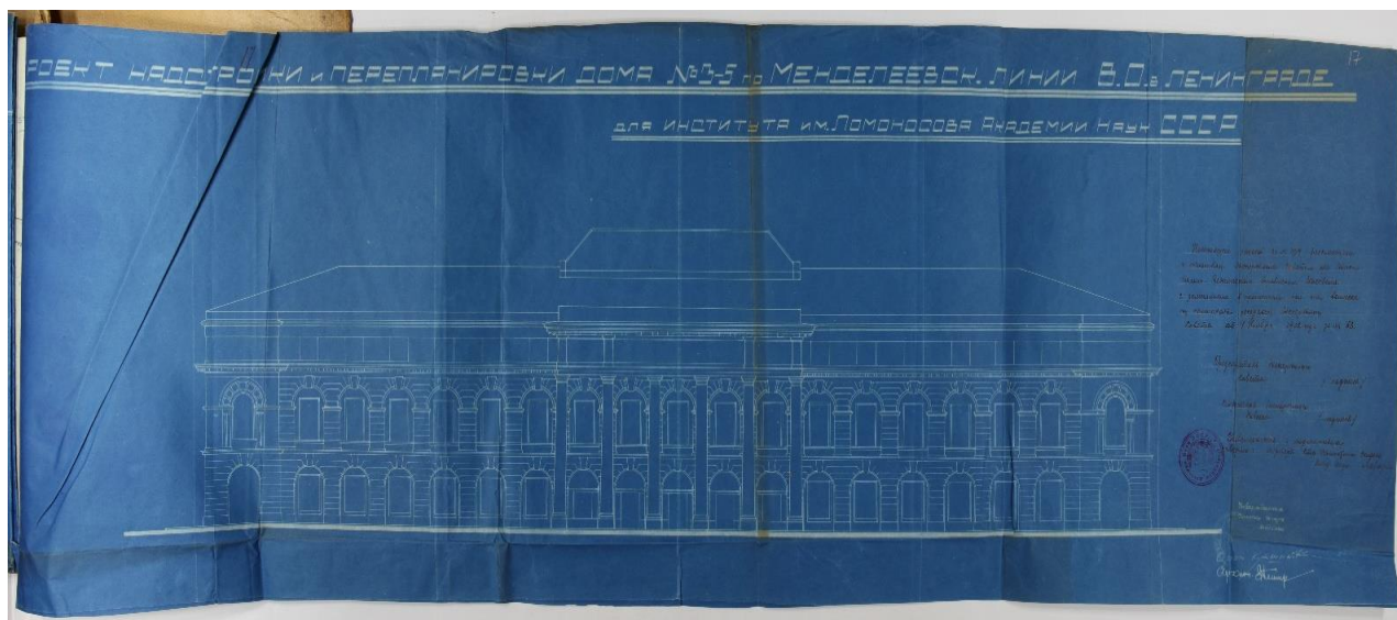
Рисунок 1. Проект надстройки и перестройки дома № 3-5 по Менделеевской линии Васильевского острова в Ленинграде [3, Л. 17].
