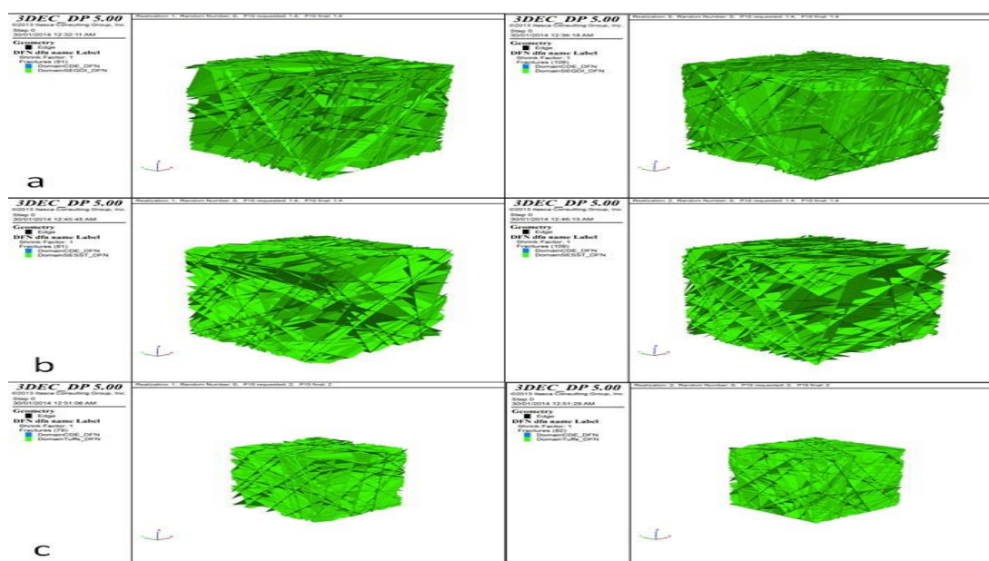
Рисунок 1.2 Примеры СДТ: (а) кварцевых диоритов, (b) отложений и (c) туфов.
