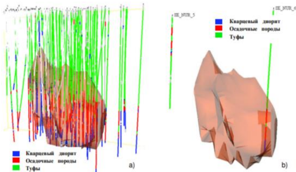
Рисунок 1.1 Примеры ДСТ построенные для интрузивной брекчии (a) и кварцевого диорита (b)
