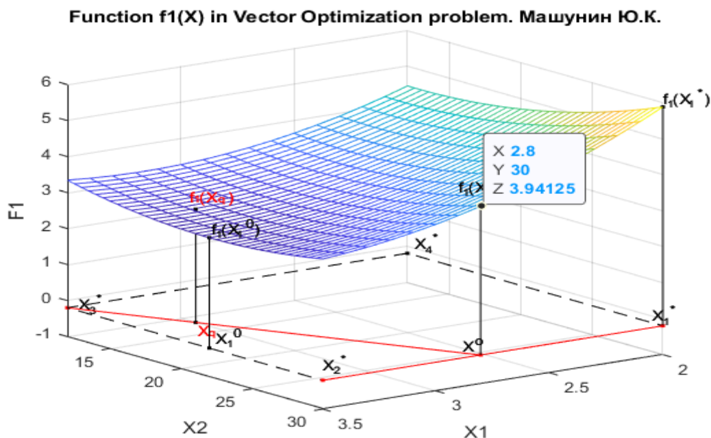
Рис. 7.5. Геометрическая интерпретация f_1(X) технологического процесса в физических показателях.
