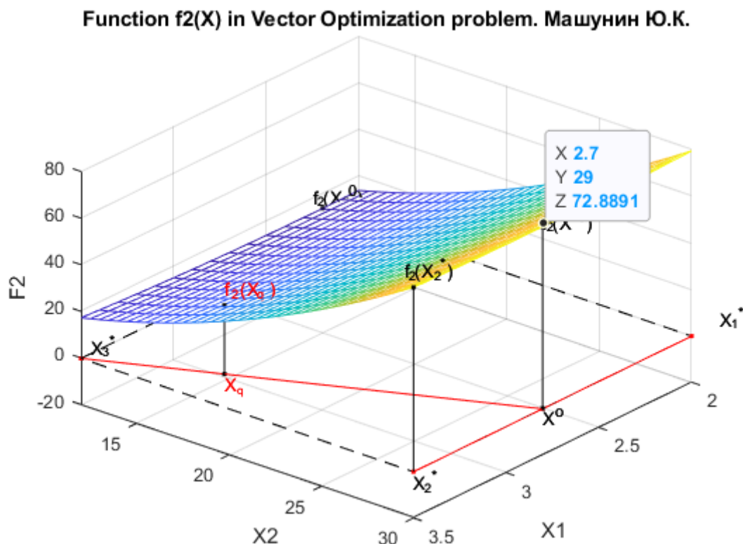
Рис. 7.6. Геометрическая интерпретация второй характеристики f_2(X) технологического процесса в физических показателях
