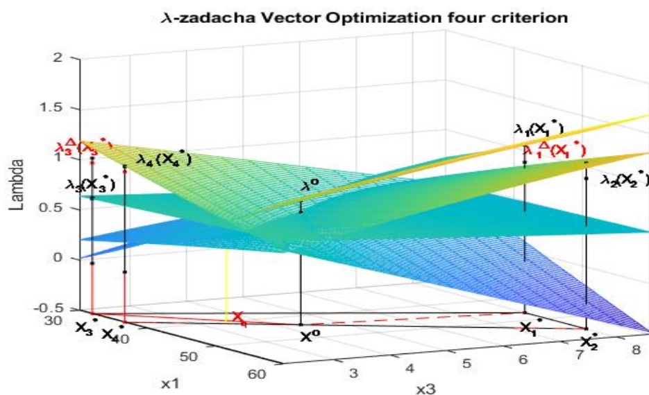
Рис. 6.2. Решение \lambda -задачи в трехмерной системе координат x_1, x_3 (= y_1, y_3), \lambda
