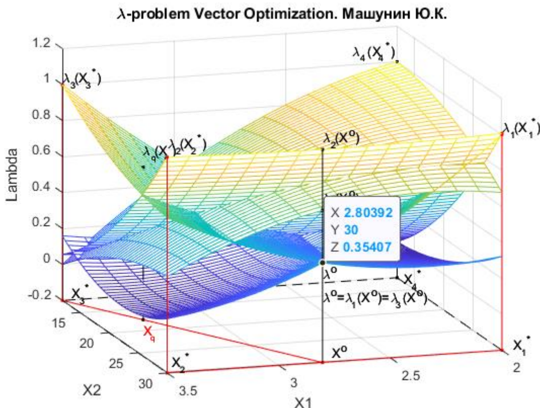
Рис. 7.2. Геометрическая интерпретация решения \lambda -задачи \lambda_1(Y), \lambda_2(Y), \lambda_3(Y), \lambda_4(Y) в трехмерной системе координат x_1, x_2 и \lambda
