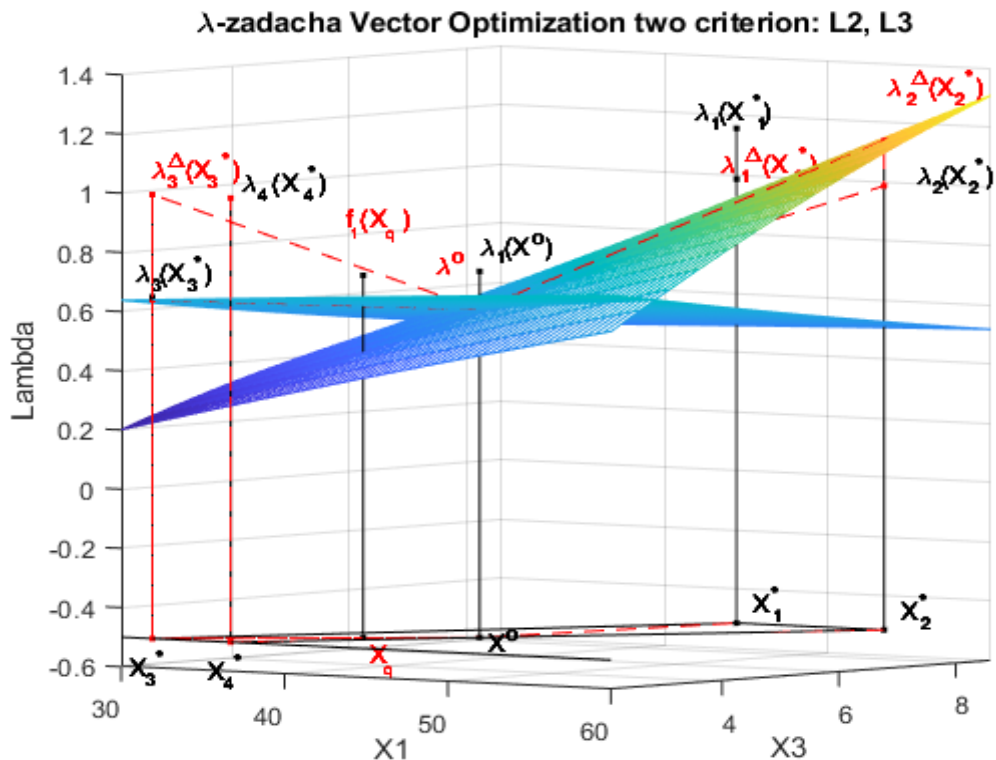
Рис. 6.5. Функции \lambda_2(X) , \lambda_3(X) и \lambda^0 в \lambda -задаче в двухмерной системе координат x_1 x_3 и \lambda и геометрическая интерпретация \lambda_2(X) , \lambda_3(X) в четырех мерной системе координат x_1 x_2 x_3 x_4
