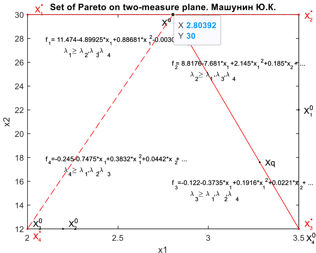
Рис. 7.1. Множество Парето, S^0 \subset S , точки оптимума X_1^*, X_2^*, X_3^*, X_4^* , и оптимальная точка X^0 в двухмерной системе координат \{x_1, x_2\} .
