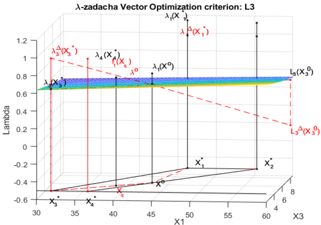
Рис. 6.7. Функции \lambda_3(X) и \lambda^0 в \lambda -задаче в двухмерной системе координат x_1 x_3 и \lambda и геометрическая интерпретация \lambda_3(X) в четырех мерной системе координат x_1 x_2 x_3 x_4 , (выделено красным цветом).
