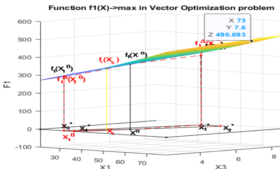
Рис. 6.8. Функция f_1(X) в двухмерной системе координат x_1, x_3 и геометрическая интерпретация функции f_1(X) в системе координат x_1, x_2, x_3, x_4
