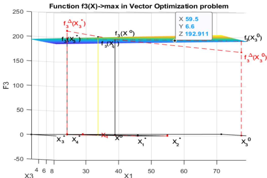
Рис. 6.10. Функция f_3(X) в двухмерной системе координат x_1, x_3 и геометрическая интерпретация функции f_3(X) в системе координат x_1, x_2, x_3, x_4
