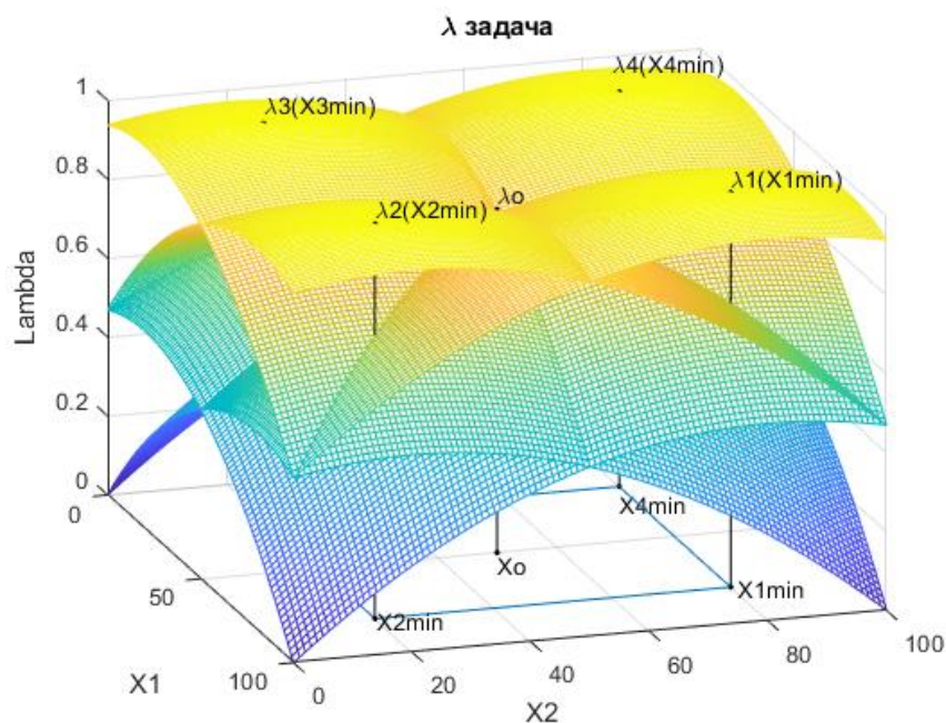
Рис. 5.2. Функции \lambda_1(X), \lambda_2(X), \lambda_3(X), \lambda_4(X) , точки оптимума X^o и \lambda^o .
