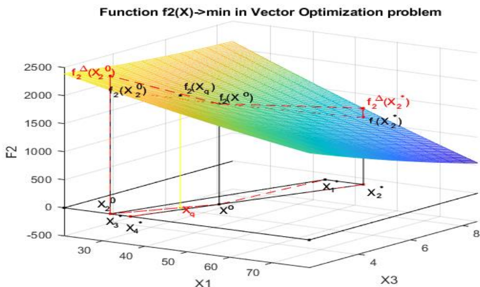
Рис. 6.9. Функция f_2(X) в двухмерной системе координат x_1, x_3 и геометрическая интерпретация функции f_2(X) в системе координат x_1, x_2, x_3, x_4
