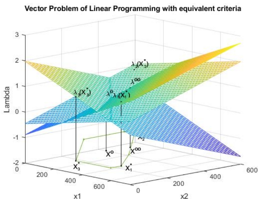
Рис. 3.4. Функции \lambda_1(X), \lambda_2(X), \lambda_3(X) и точки оптимума X^o и \lambda^o
