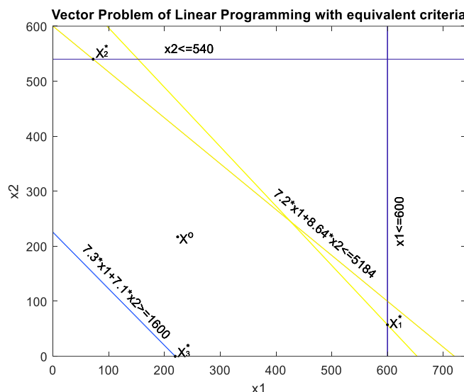
Рис. 5.1. Допустимое множество решений ВЗЛП (3.14)- (3.17) и результаты решения
