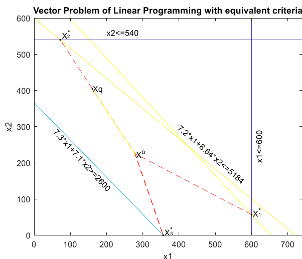
Рис. 3.5. Допустимое множество точек (3.25)- (3.27), точки оптимума X_1^* , X_2^* and X_3^* , точка оптимума X^0 и точка оптимума X^q , полученная при приоритете критерия q = 2 .
