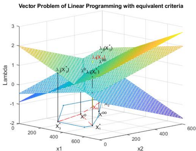
Рис. 3.6. Функции \lambda_1(X) , \lambda_2(X) , \lambda_3(X) , точки оптимума X^0 и \lambda^0 и точка оптимума X^q , полученная при приоритете критерия q = 2
