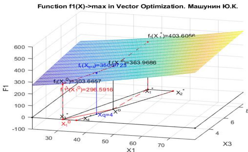
Рис. 6k4. Функция f_1(X) с приоритетом четвертого критерия в двухмерной системе координат x_1 x_3 и геометрическая интерпретация функции f_1(X) в системе координат x_1 x_2 x_3 x_4
