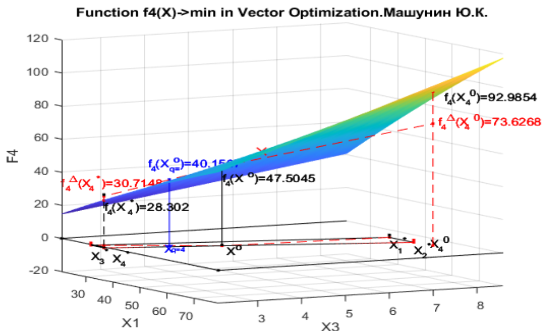
Рис. 9.k4. Функция f_4(X) с приоритетом четвертого критерия в двухмерной системе координат x_1 x_3 и геометрическая интерпретация функции f_4(X) в системе координат x_1 x_2 x_3 x_4
