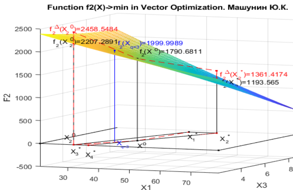
Рис. 7.k3. Функция f_2(X) с приоритетом третьего критерия в двухмерной системе координат x_1, x_3 и геометрическая интерпретация функции f_2(X) в системе координат x_1, x_2, x_3, x_4
