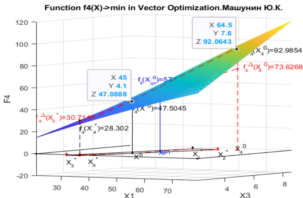
Рис. 9.k1. Функция f_4(X) в двухмерной системе координат x_1, x_3 и геометрическая интерпретация функции f_4(X) с приоритетом первого критерия в системе координат x_1, x_2, x_3, x_4
