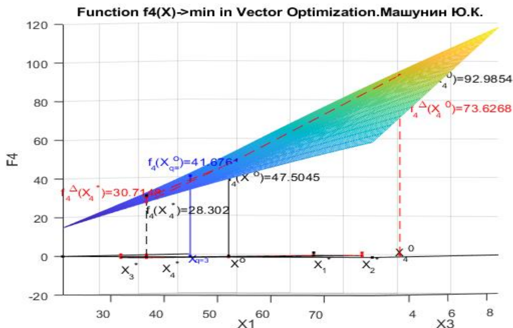
Рис. 9.k3. Функция f_4(X) с приоритетом третьего критерия в двухмерной системе координат x_1 x_3 и геометрическая интерпретация функции f_4(X) в системе координат x_1 x_2 x_3 x_4
