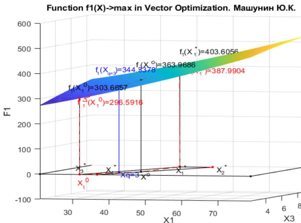
Рис. 6.k3. Функция f_1(X) с приоритетом третьего критерия в двухмерной системе координат x_1 x_3 и геометрическая интерпретация функции f_1(X) в системе координат x_1 x_2 x_3 x_4
