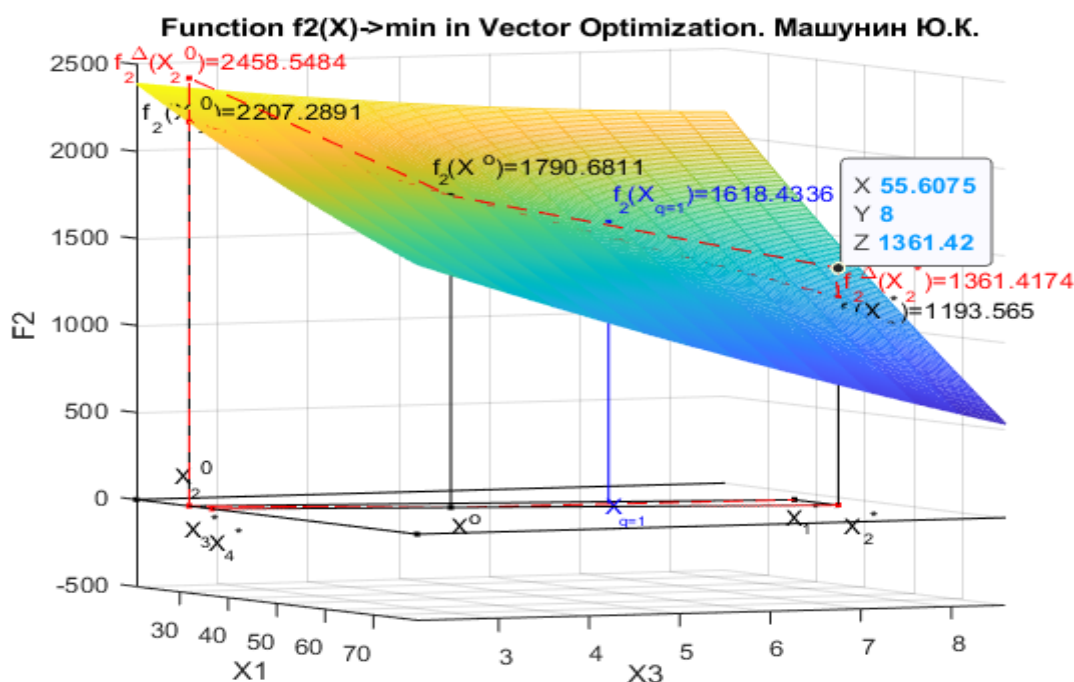
Рис. 7.k1. Функция f_2(X) с приоритетом первого критерия в двухмерной системе координат x_1, x_3 , геометрическая интерпретация функции f_2(X) - координаты x_1, x_2, x_3, x_4
