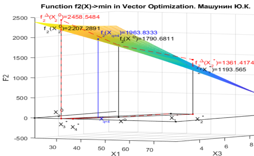
Рис. 7.k4. Функция f_2(X) с приоритетом четвертого критерия в двухмерной системе координат x_1, x_3 и геометрическая интерпретация функции f_2(X) в системе координат x_1, x_2, x_3, x_4
