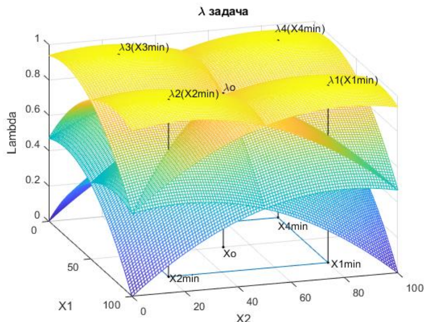
Рис. 5.2. Функции \lambda_1(X), \lambda_2(X), \lambda_3(X), \lambda_4(X) , точки оптимума X^o и \lambda^o .
