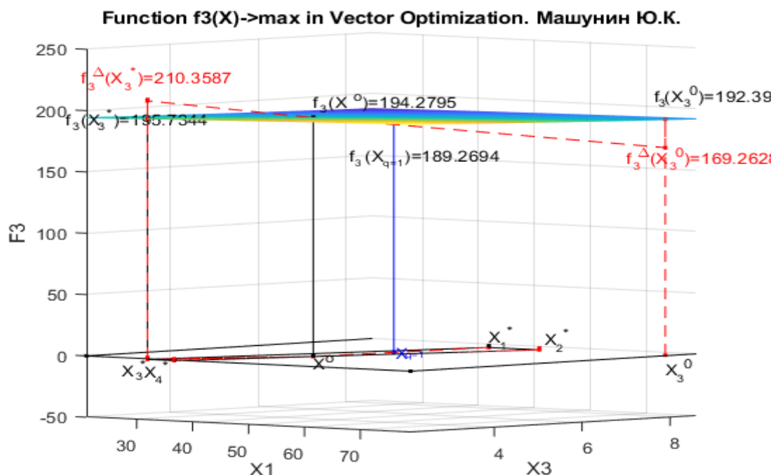
Рис. 8.k1. Функция f_3(X) с приоритетом первого критерия в двухмерной системе координат x_1, x_3 , геометрическая интерпретация функции f_3(X) в системе координат x_1, \dots, x_4 .
