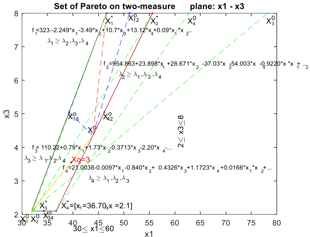
Рис. 1. Допустимое множество точек S в координатах x_1, x_3 . Множество точек, оптимальных по Парето, S^0 \subset S , ограничено точками X_1^*, X_2^*, X_3^*, X_4^* , и локальное S_1^0 между X_1^*, X_{13}^0, X^0, X_{12}^0, X_1^* в двухмерной системе координат \{x_1, x_3\} .
