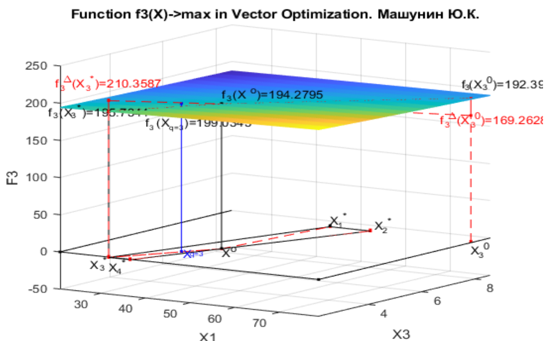
Рис. 8.k3. Функция f_3(X) с приоритетом третьего критерия в двухмерной системе координат x_1, x_3 и геометрическая интерпретация функции f_3(X) в системе координат x_1, x_2, x_3, x_4
