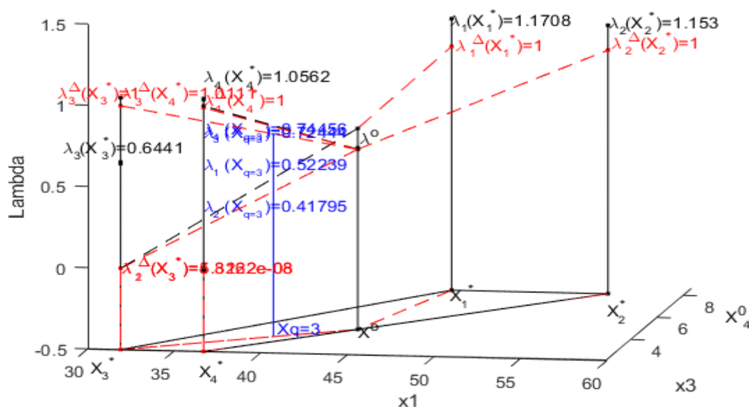
Рис. 5к3. \lambda -задача в системе координат x_1 x_3 (= y_1 y_3) и \lambda . Результаты решения: \lambda_k^\Delta(X_k^*) = 1, k = \overline{1, K} ; относительные оценки с приоритетом третьего критерия в точке оптимума X_{q=3} : \lambda_k(X_{q=3}), k = \overline{1, K} .
