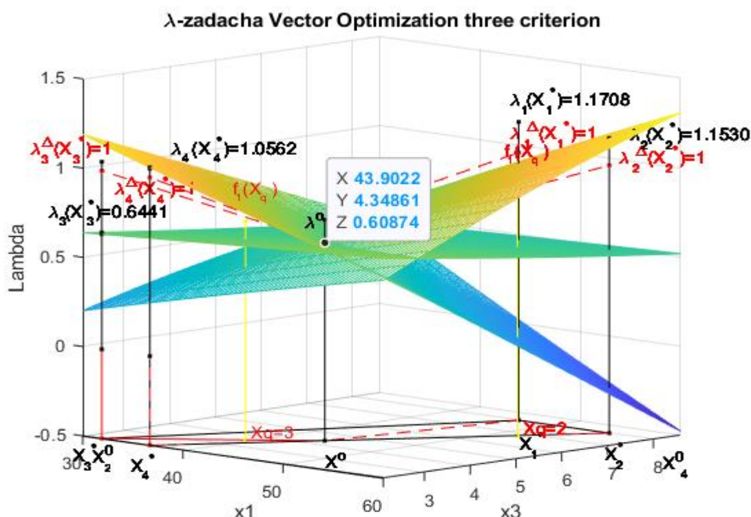
Рис. 3. Решение \lambda -задачи в трехмерной системе координат x_1, x_3 ( = y_1, y_3 ) и \lambda
