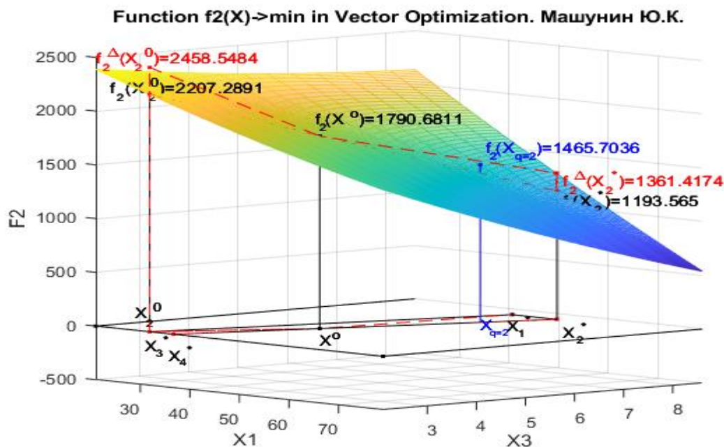
Рис. 9. Функция f_2(X) с приоритетом второго критерия в двухмерной системе координат x_1, x_3 и геометрическая интерпретация функции f_2(X) в системе координат x_1, x_2, x_3, x_4
