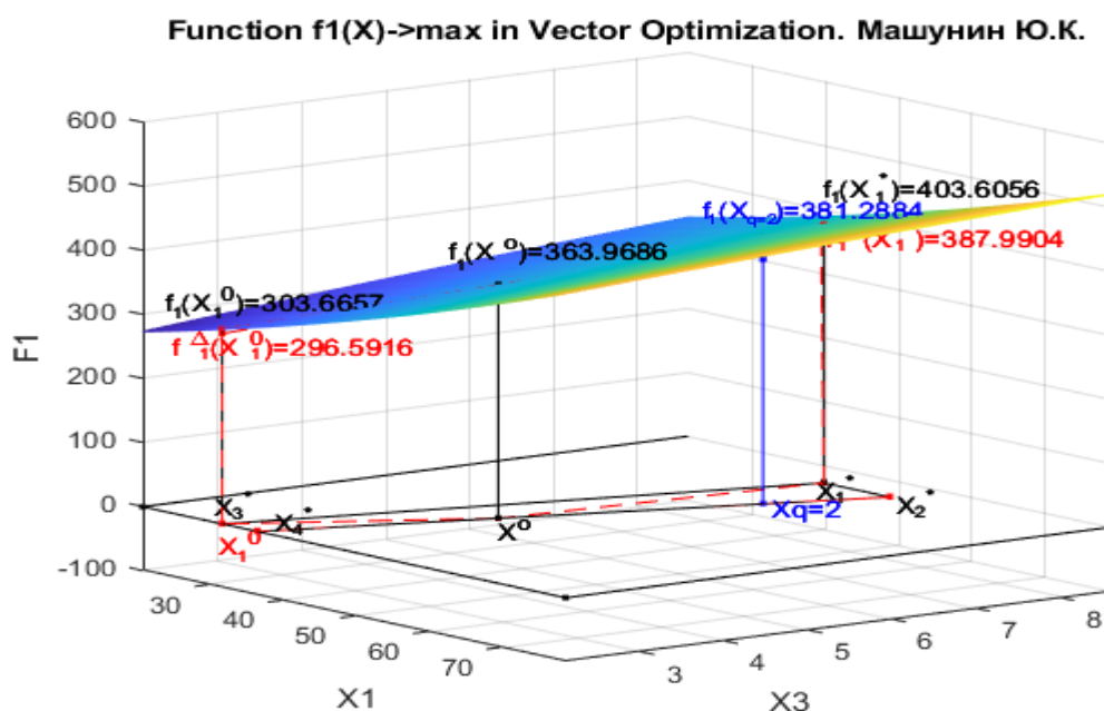
Рис. 6k2. Функция f_1(X) с приоритетом второго критерия в двухмерной системе координат x_1, x_3 и геометрическая интерпретация функции f_1(X) в системе координат x_1, x_2, x_3, x_4
