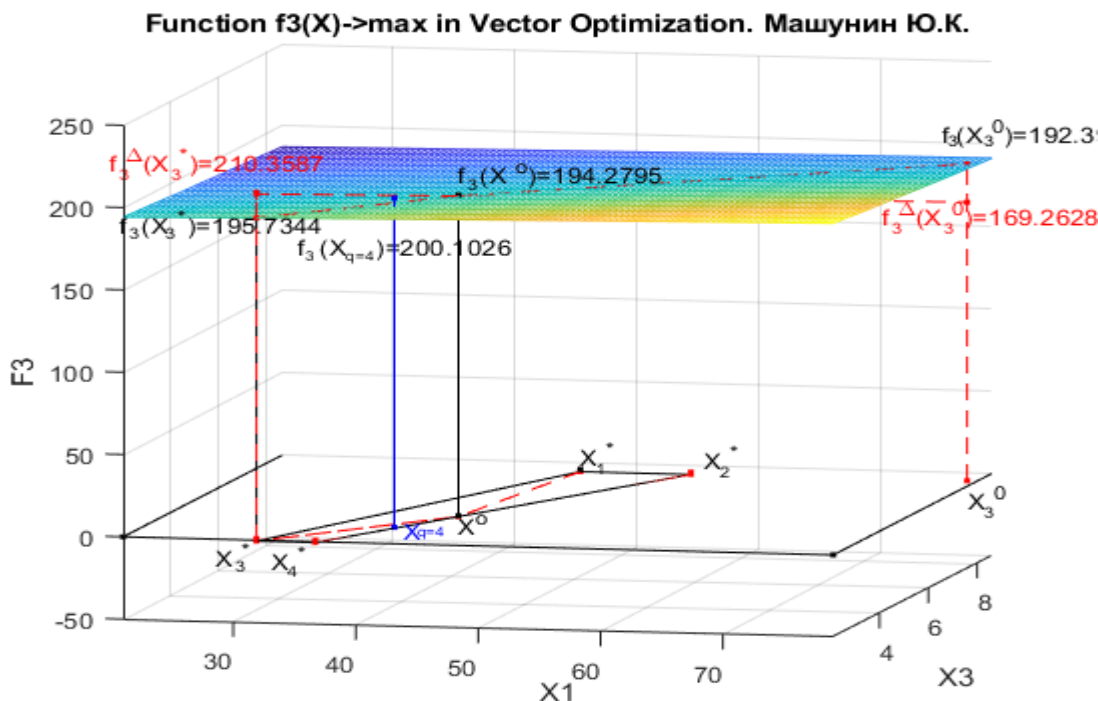
Рис. 8.k4. Функция f_3(X) с приоритетом четвертого критерия в двухмерной системе координат x_1, x_3 и геометрическая интерпретация функции f_3(X) в системе координат x_1, x_2, x_3, x_4
