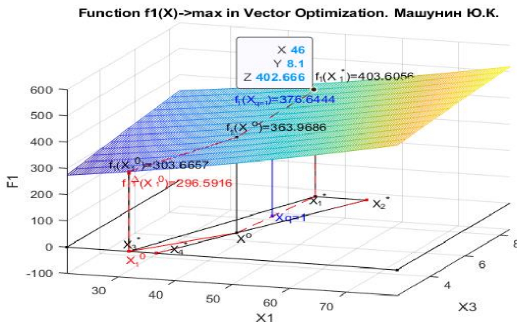
Рис. 6k1. Функция f_1(X) с приоритетом первого критерия в двухмерной системе координат x_1 x_3 и геометрическая интерпретация функции f_1(X) в системе координат x_1 x_2 x_3 x_4
