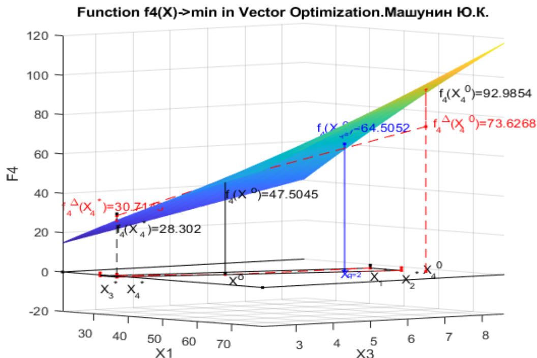
Рис. 9.k2. Функция f_4(X) с приоритетом второго критерия в двухмерной системе координат x_1, x_3 и геометрическая интерпретация функции f_4(X) в системе координат x_1, x_2, x_3, x_4
