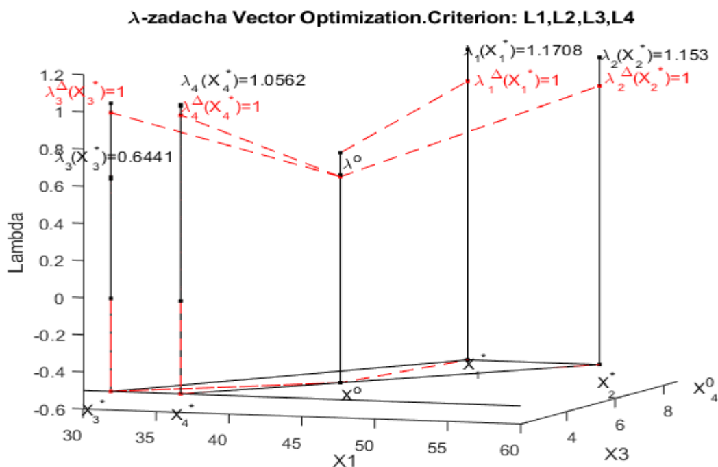
Рис. 4. \lambda -задача в системе координат x_1 x_3 ( = y_1 y_3 ) и \lambda . Результаты решения \lambda_1(Y_1^*) = \lambda_2(Y_2^*) = \lambda_3(Y_3^*) = \lambda_4(Y_4^*) = 1 ; L(Y_2^*) = \{\lambda_1(Y_2^*), \lambda_2(Y_2^*), \lambda_3(Y_2^*), \lambda_4(Y_2^*)\}
