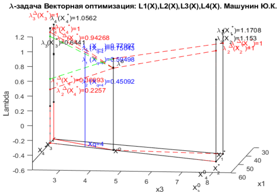
Рис. 5к3. \lambda -задача в системе координат x_1 x_3 (= y_1 y_3) и \lambda . Результаты решения: \lambda_k^A(X_k^*) = 1, k = \overline{1, K} ; относительные оценки с приоритетом четвертого критерия в точке оптимума X_{q=4} : \lambda_k(X_{q=4}), k = \overline{1, K} .
