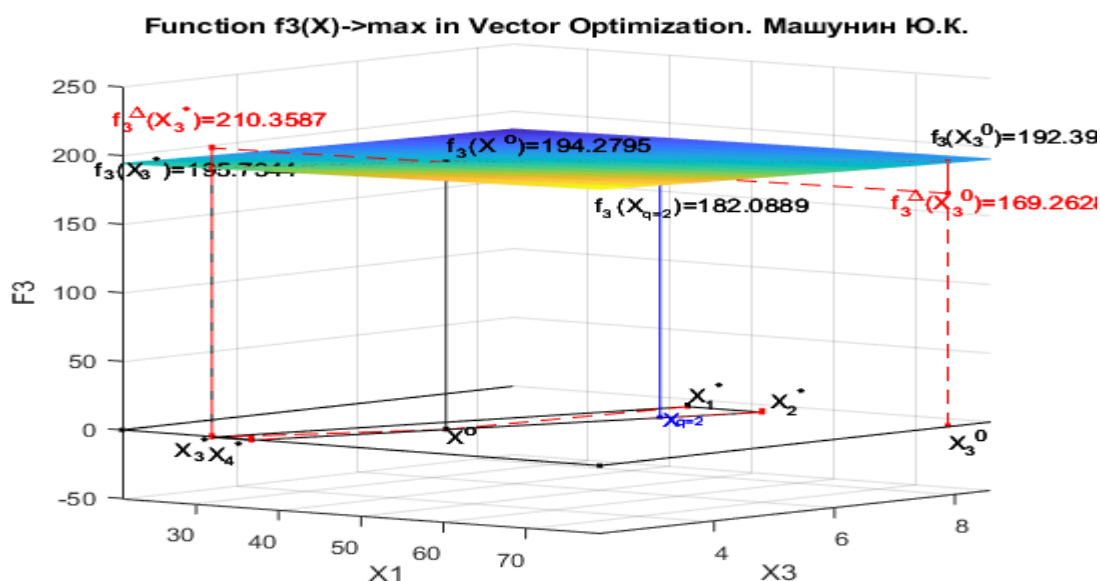
Рис. 8.k2. Функция f_3(X) с приоритетом второго критерия в двухмерной системе координат x_1, x_3 и геометрическая интерпретация функции f_3(X) в системе координат x_1, x_2, x_3, x_4
