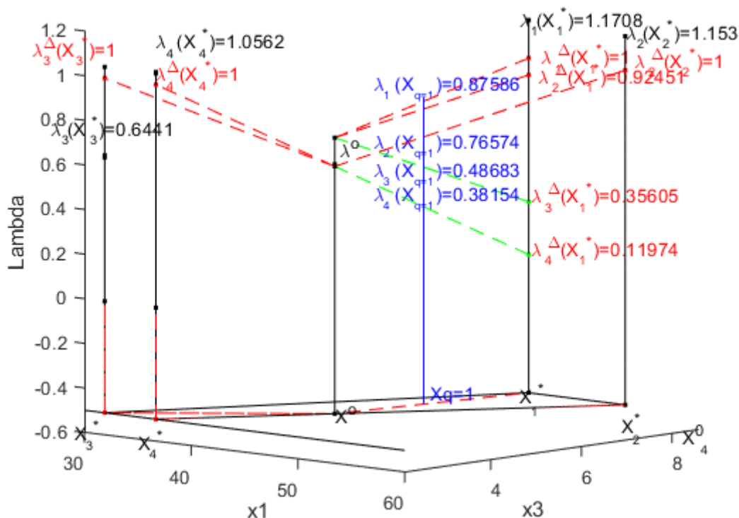
Рис. 5k1. \lambda -задача в системе координат x_1, x_3 (= y_1, y_3) и \lambda .
