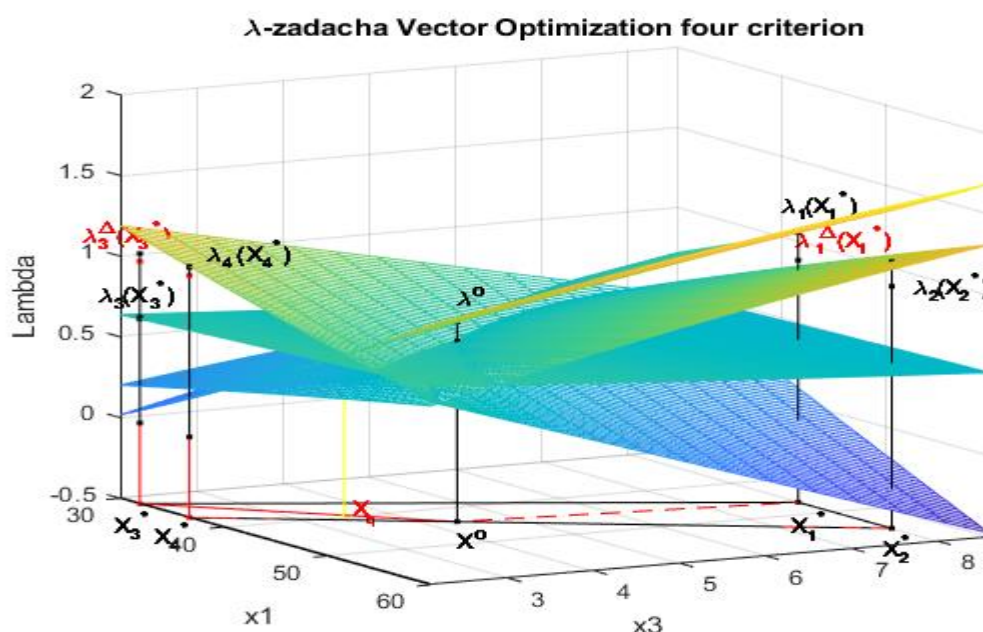
Рис. 6.2. Решение \lambda -задачи в трехмерной системе координат x_1 \ x_3 (= y_1 \ y_3) , \lambda
