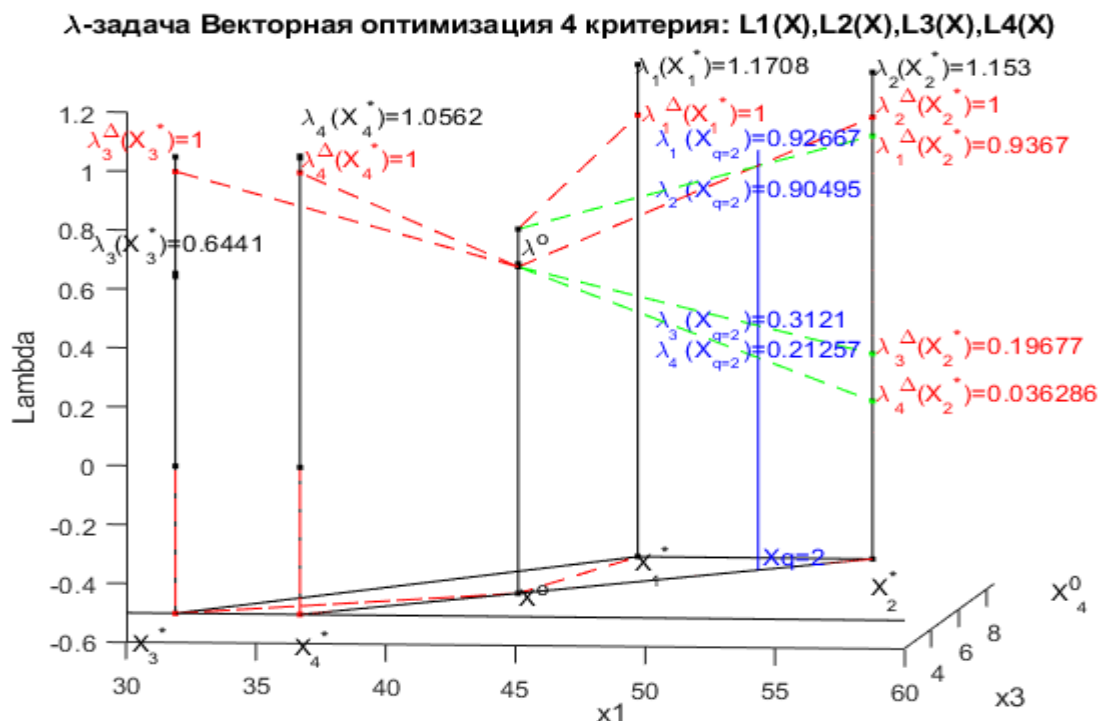
Рис. 5k2. \lambda -задача в системе координат x_1 \ x_3 (= y_1 \ y_3) и \lambda . Результаты решения: \lambda_k^A(X_k^*) = 1, k = \overline{1, K} ; относительные оценки с приоритетом второго критерия в точке оптимума X_{q=2}: \lambda_k(X_{q=2}), k = \overline{1, K} .
